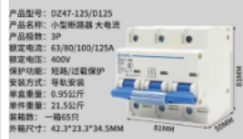
Interruptor miniatura MCB - 3P
